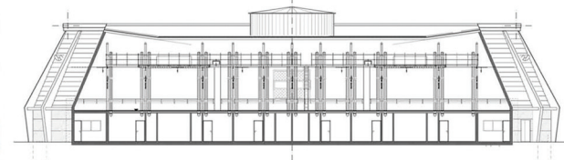
Schnitt Sanitärbereich
